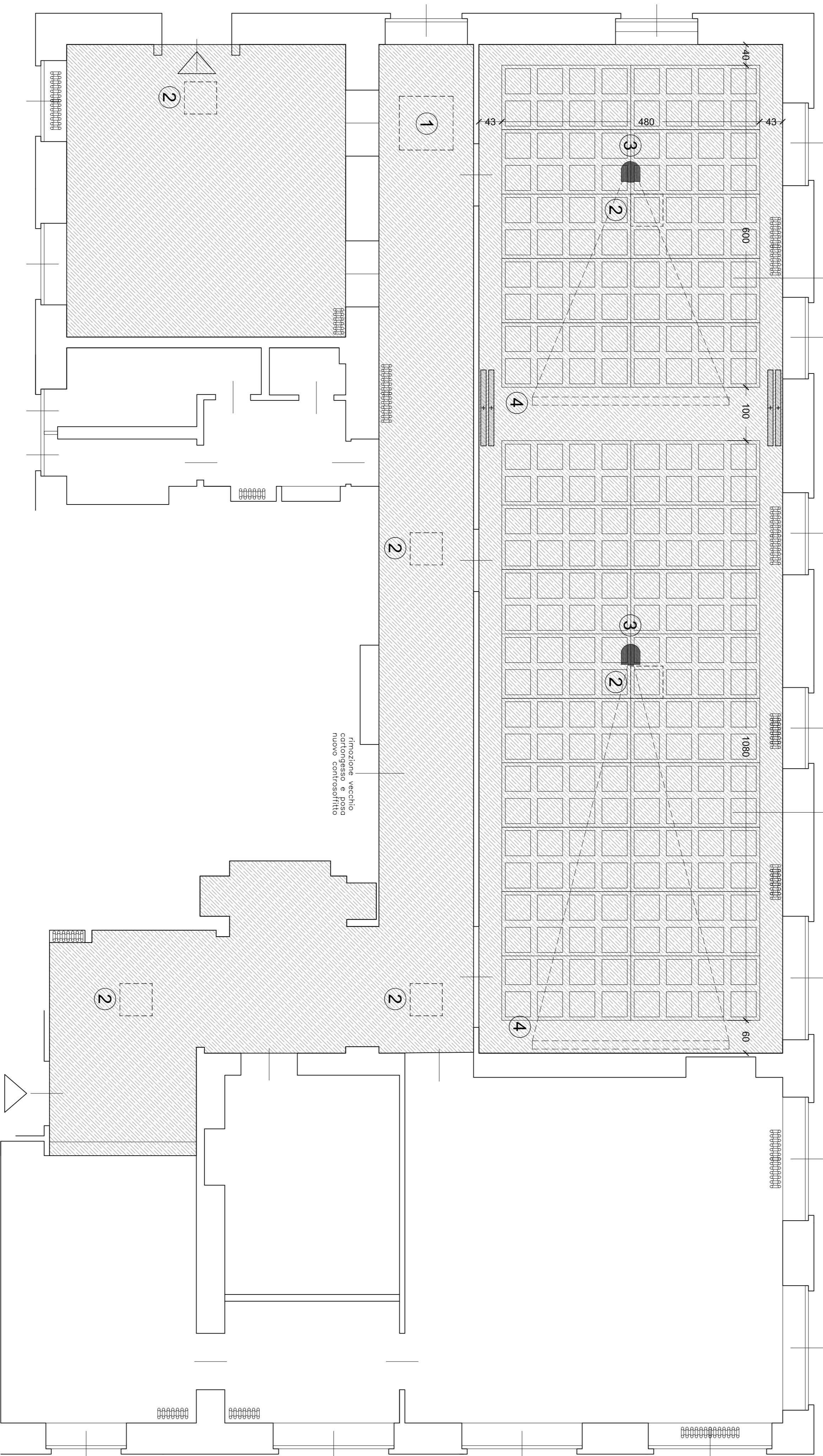
PIANTA - SCALA 1:50
