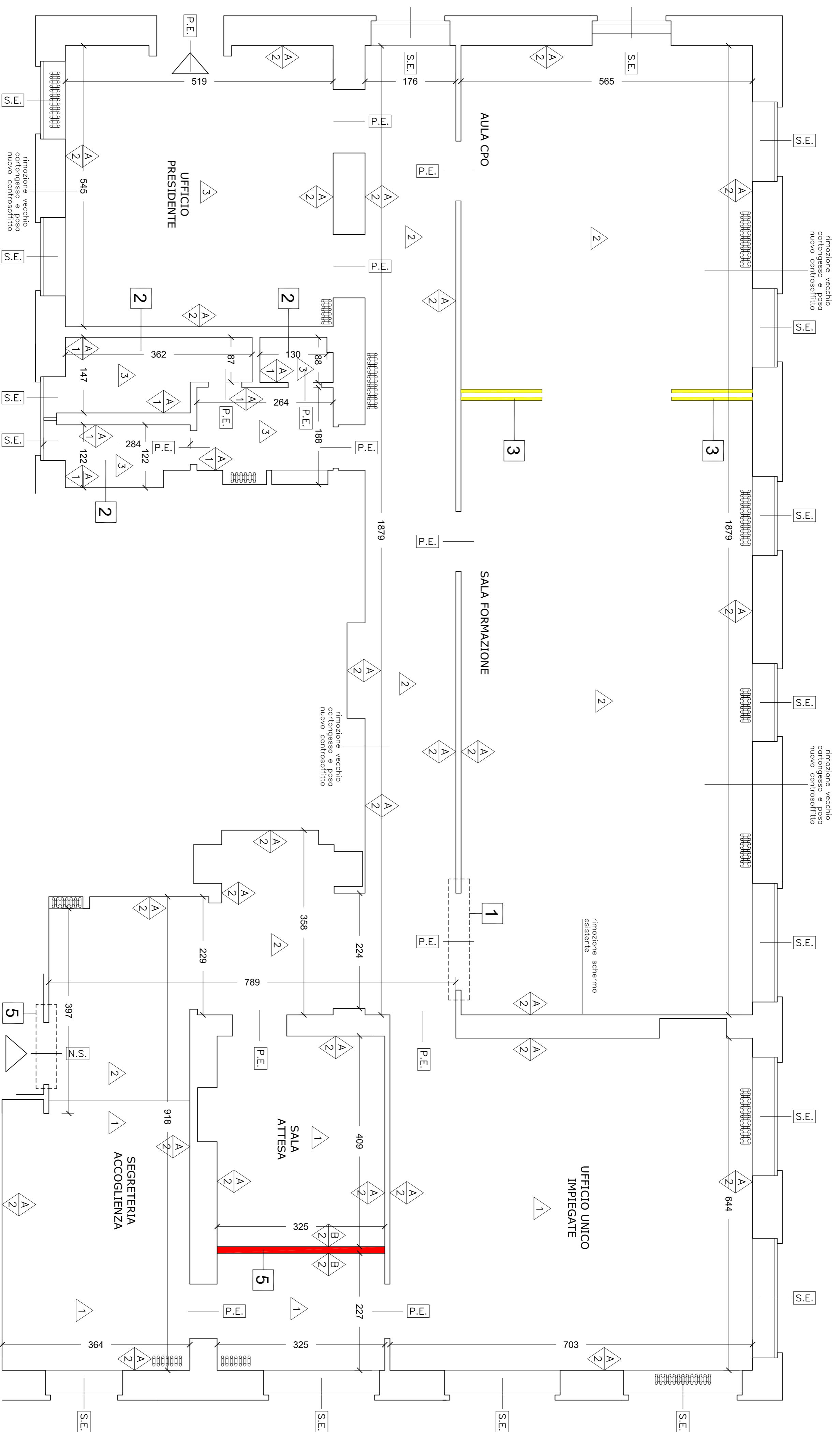
PIANTA - SCALA 1:50
